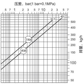
2022 型疏水阀排量图
